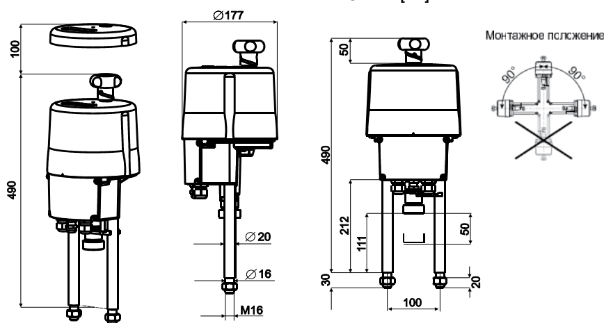
Размеры для стандартного PS-сцепления (Для вентильного шпинделя с резьбой, защищенно стопорным штифтом)
