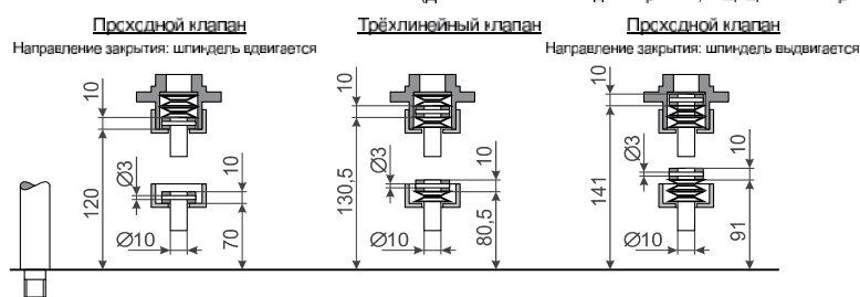
Размеры для стандартного PS-сцепления (Для вентильного шпинделя с резьбой, защищенно стопорным штифтом)
