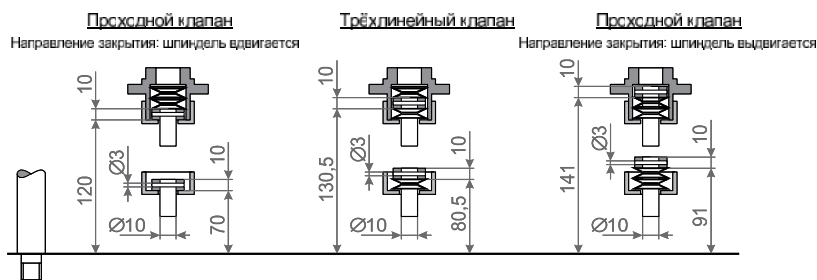
(Для вентильного шпинделя с резьбой, защищено стопорным штифтом)
